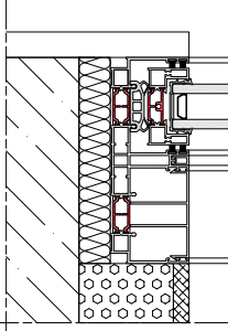
Jamb Detail
